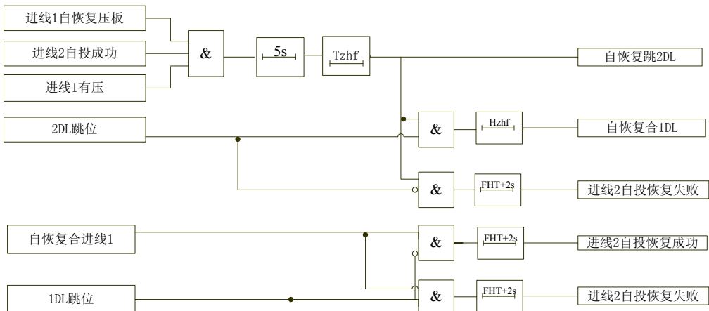
图 4-15 进线二自投自恢复逻辑图
