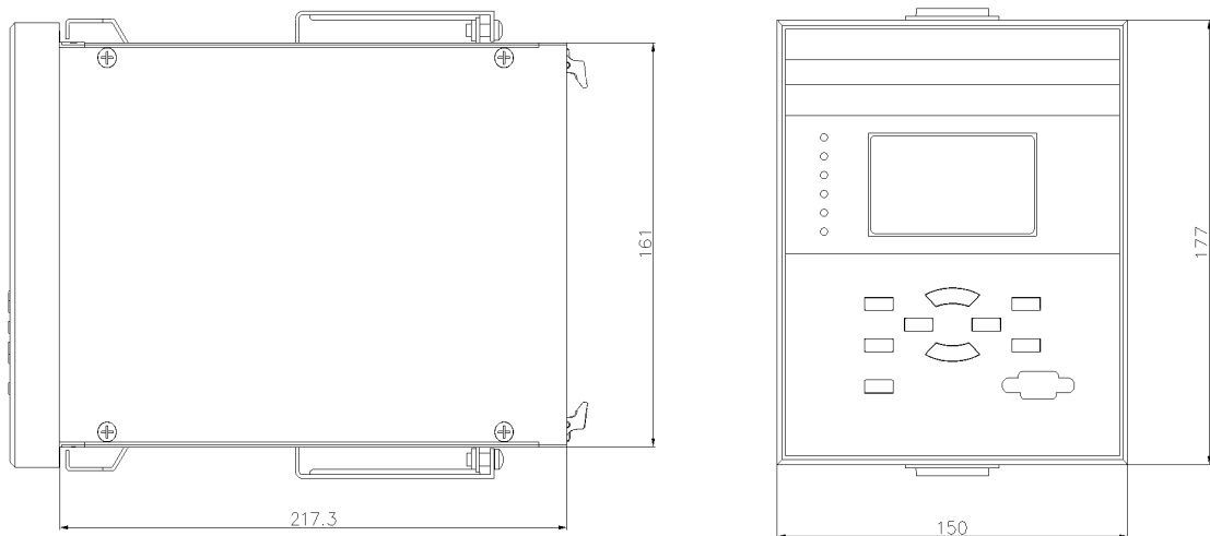
图 3-1 外形尺寸
