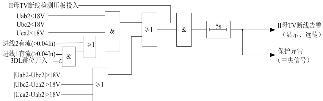
图 4-17 II 母 TV 断线告警原理
