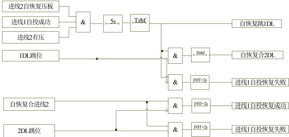
图 4-14 进线一自投自恢复逻辑图
