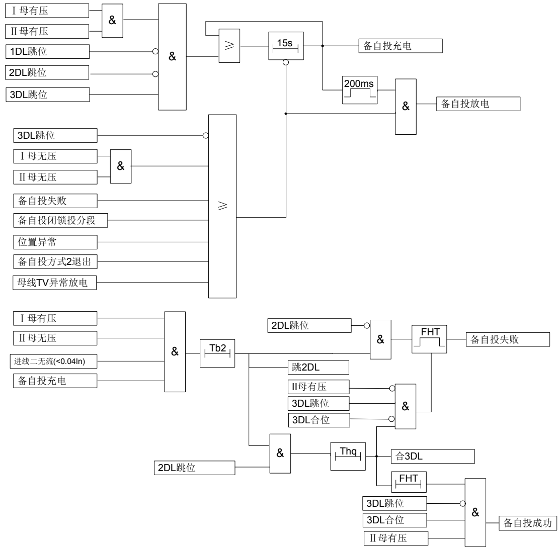
图 4-5 II 母失压自投（自投方式二）逻辑框图
