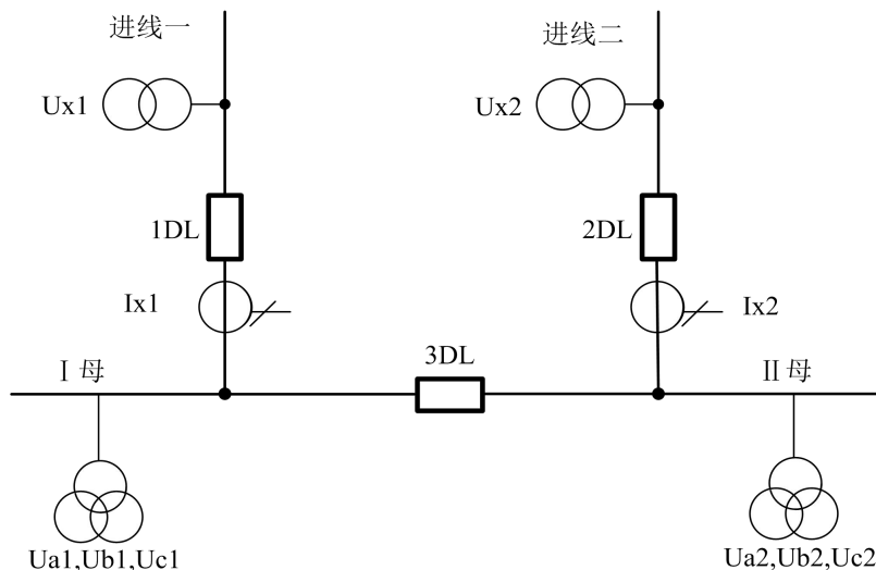
图 4-1 运行方式接线图 1
