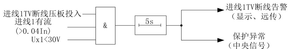
图 4-18 进线 1 TV 断线告警原理
