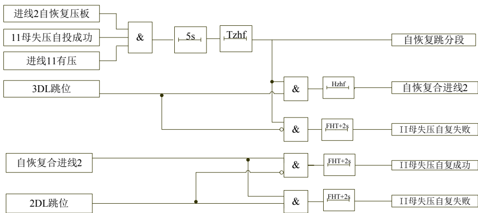
图 4-13 II 母失压自恢复逻辑图
