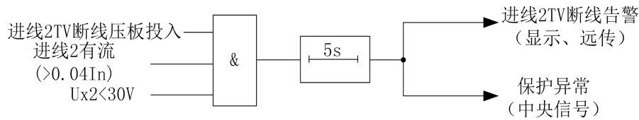
图 4-19 进线 2 TV 断线告警原理
