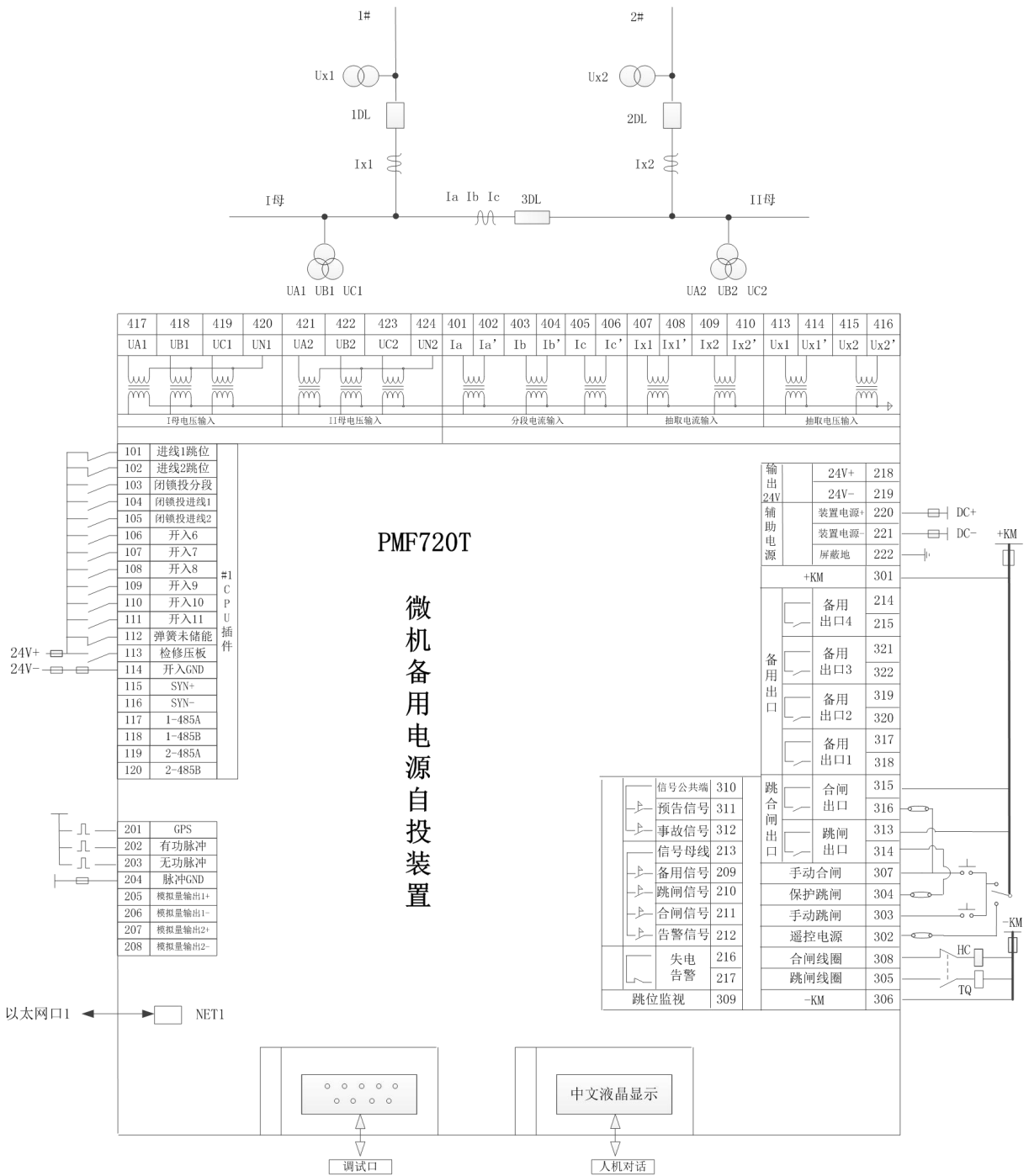
接线示意图
