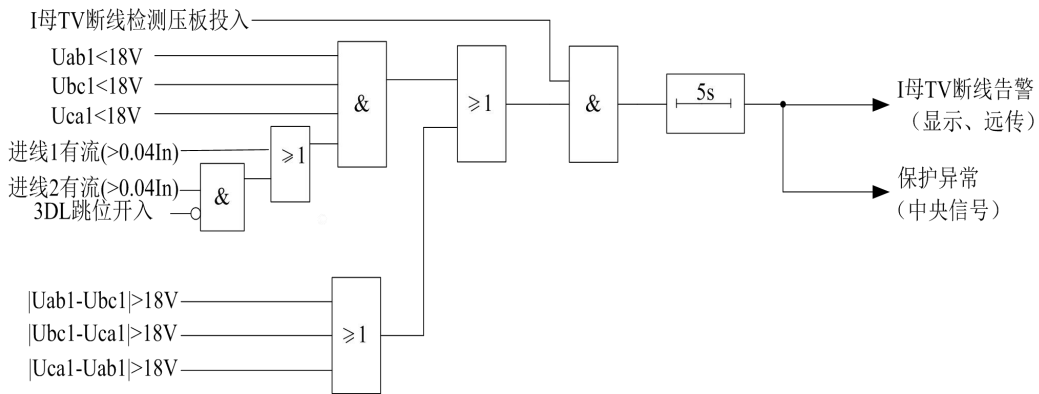
图 4-16 I 母 TV 断线告警原理
