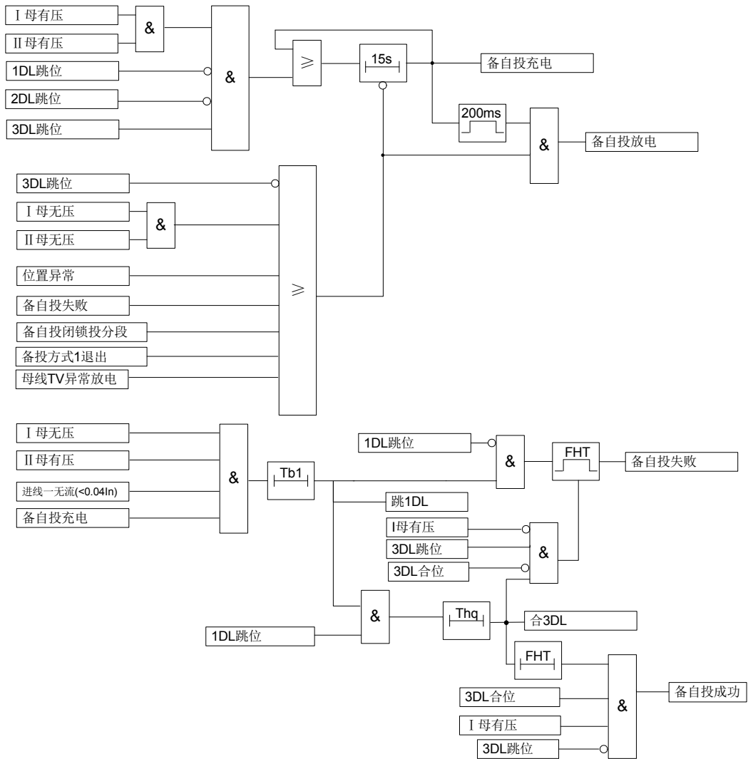
图 4-4 I 母失压自投（自投方式一）逻辑框图
