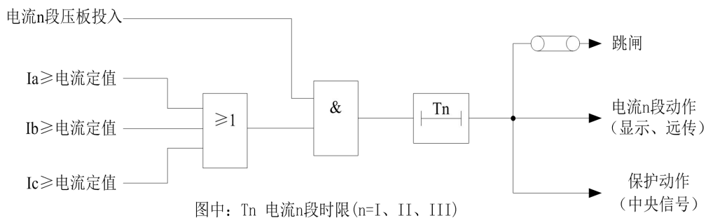
图 4-10 三段式电流保护逻辑框图
