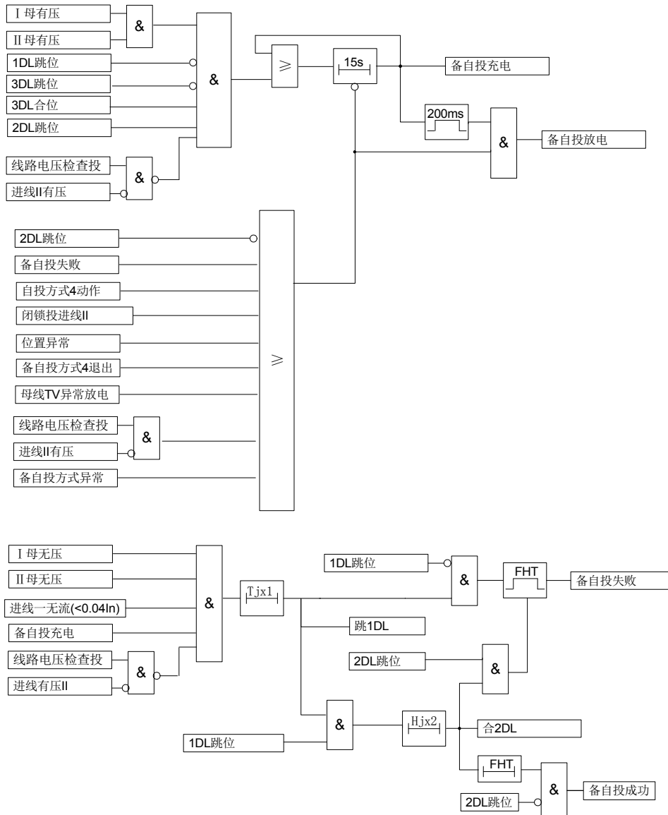
图 4-7 进线二自投（自投方式 4）逻辑框图
