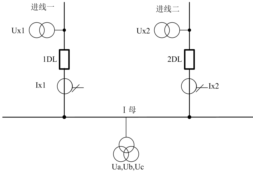
图 4-2 运行方式接线图 2
