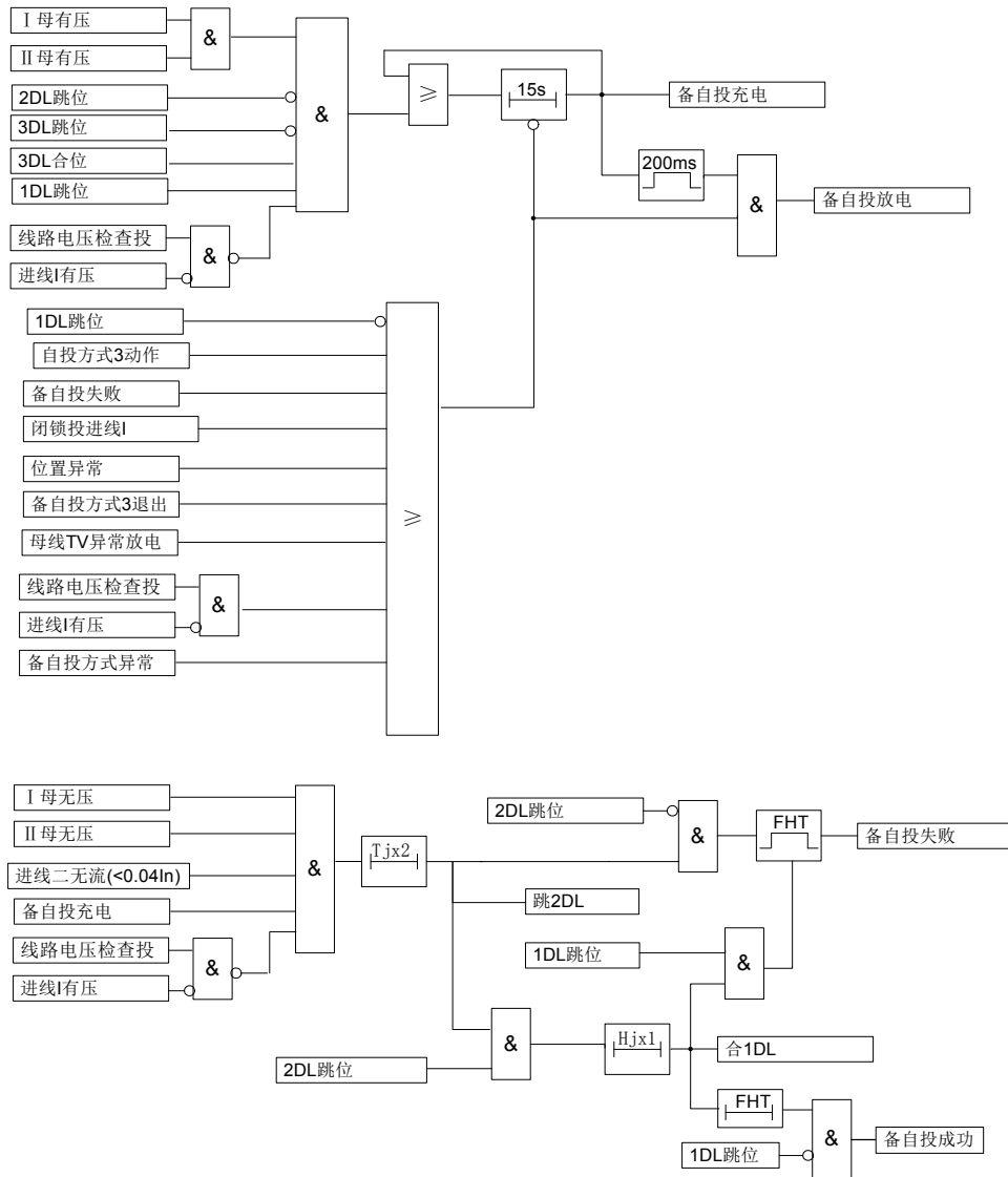
图 4-6 进线一自投（自投方式 3）逻辑框图
