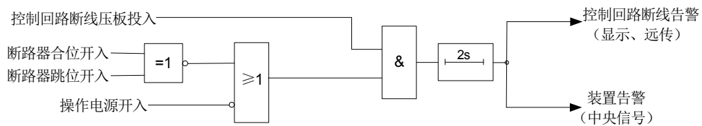
图 4-20 控制回路断线检测逻辑框
