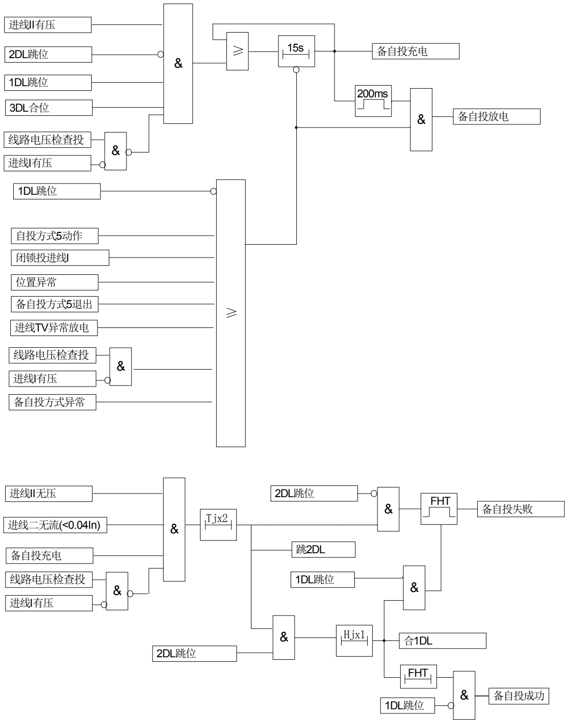
图 4-8 进线一自投（自投方式 5）逻辑框图
