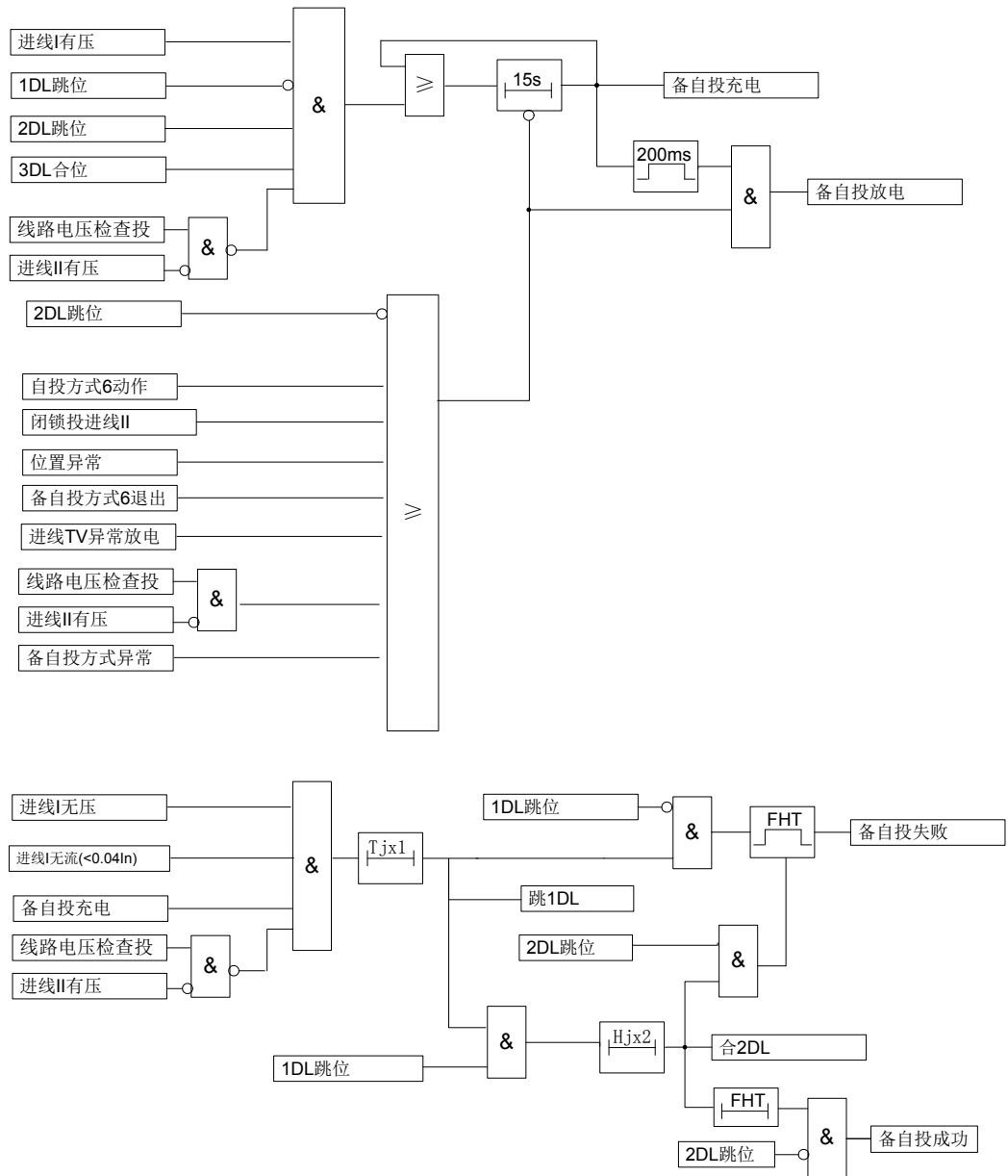
图 4-9 进线二自投（自投方式 6）逻辑框图
