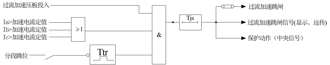
图中Ttr表示加速投入时限
