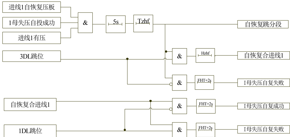
图 4-12 I 母失压自恢复逻辑图
