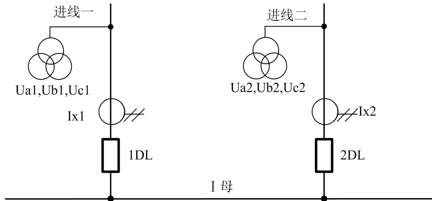
母线无PT、进线为3相PT的情况
