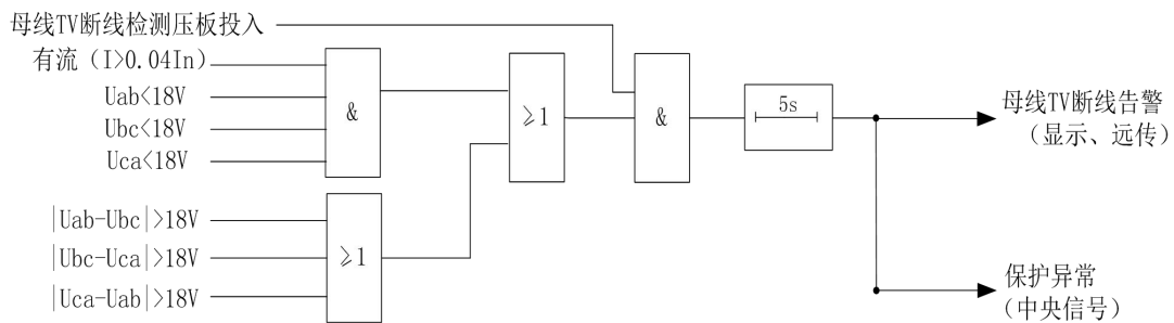
图 4-10 母线 TV 断线检测逻辑框图
