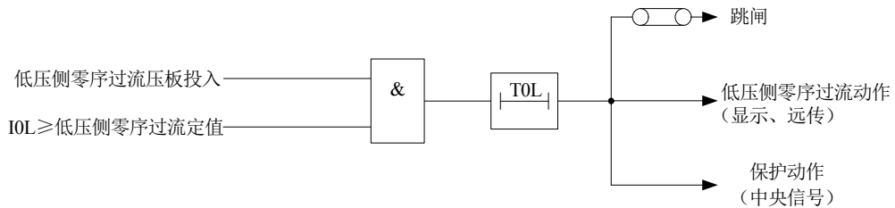
图 4-5 低压侧零序过流保护逻辑框图
