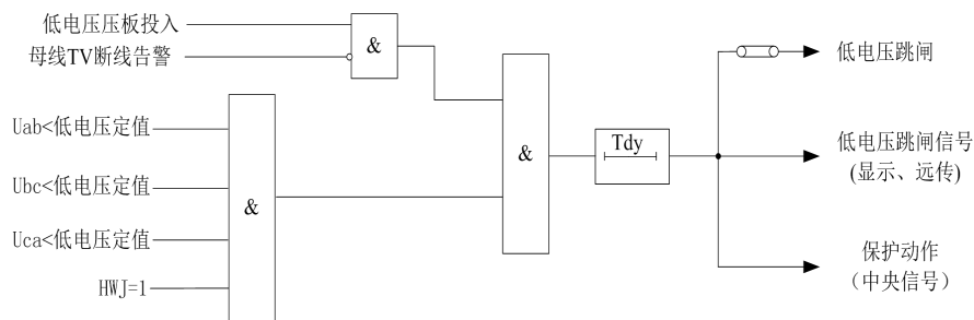
图中Tdy为低电压延时
