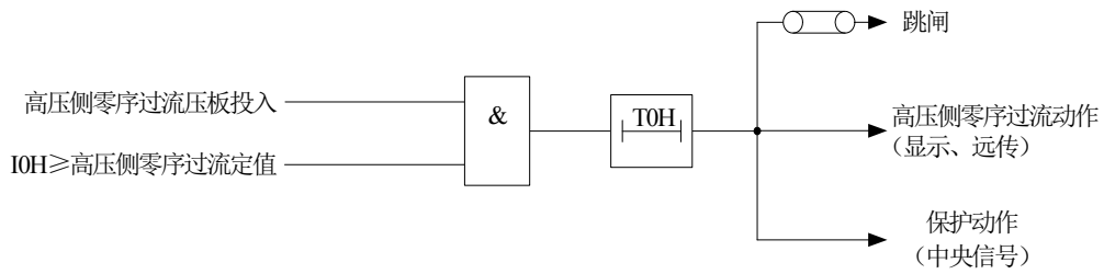
图 4-4 高压侧零序过流保护逻辑框图
