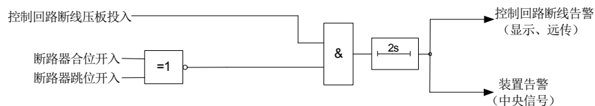
图 4-11 控制回路断线检测逻辑框图
