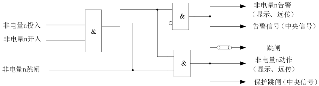
图 4-9 非电量保护逻辑框图
