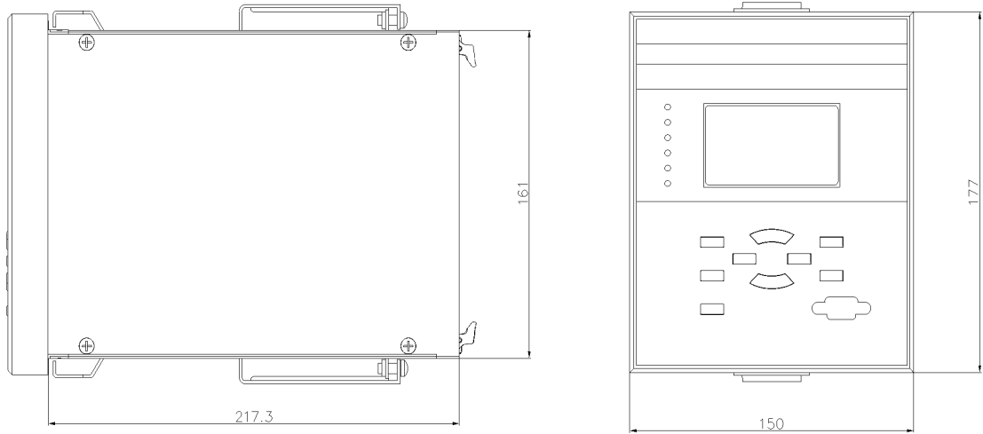
图 3-1 外形尺寸
